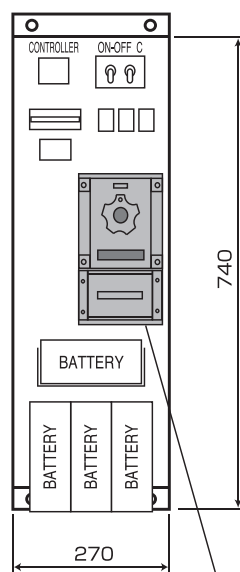
〈基板正面図〉
