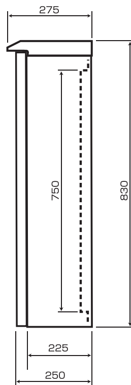
〈側面寸法図〉
