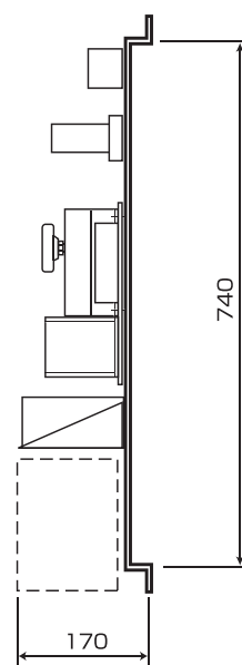
〈基板側面図〉
